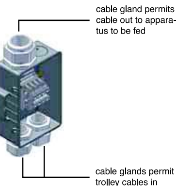
TTB70-4
