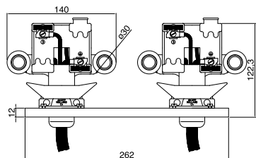
CL4-70
